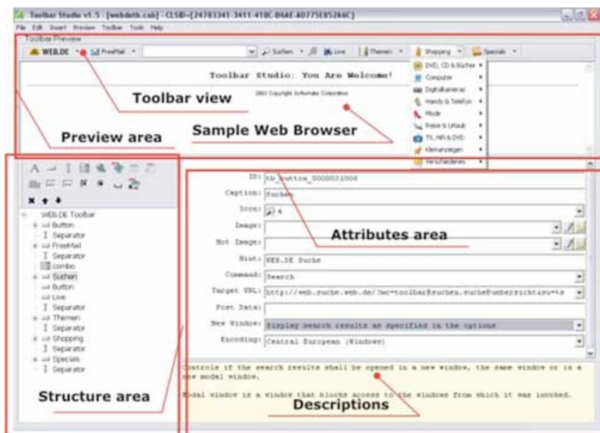
L'interface du kit de développement est simple et efficace
